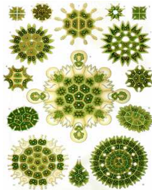
Haeckel
